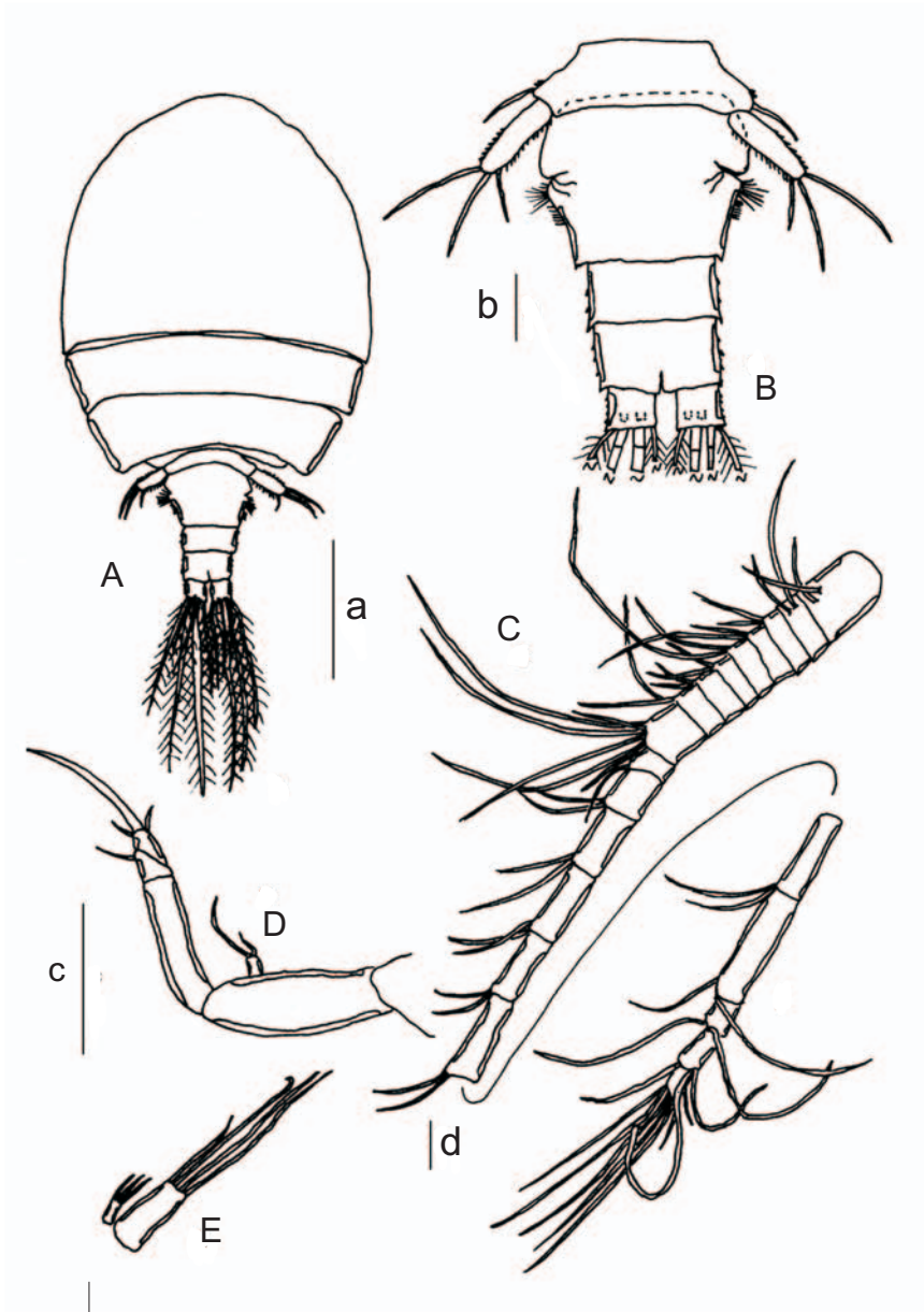
Fig. 1. Asterocheres garridoi sp. nov. Hembra A: Vista dorsal del holótipo (a); B: Vista ventral del urosoma (b); C: Anténula (c); D: Antena (d); E: Maxíla (e). Escala. a: 0.2 mm; b, d: 0.02 mm, c: 0.05 mm.
