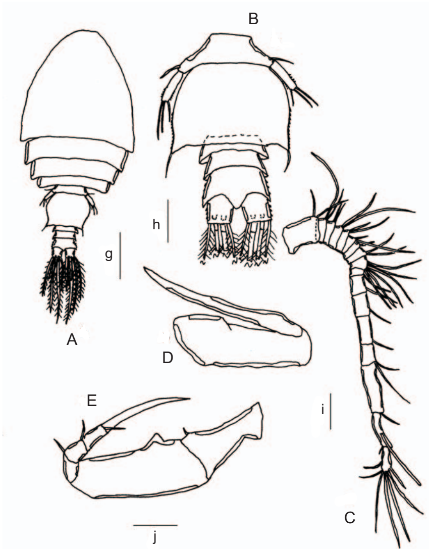
Fig. 3. Asteroberes garridoi sp. nov. Macho. A: Vista dorsal del alótipo (g); B: Vista ventral del urosoma (h); C: Anténula (i); D: Maxila (j) y E: Maxilpedo (j). Escala. g: 0.1mm; h,j: 0.2 mm, i: 0.05 mm.
