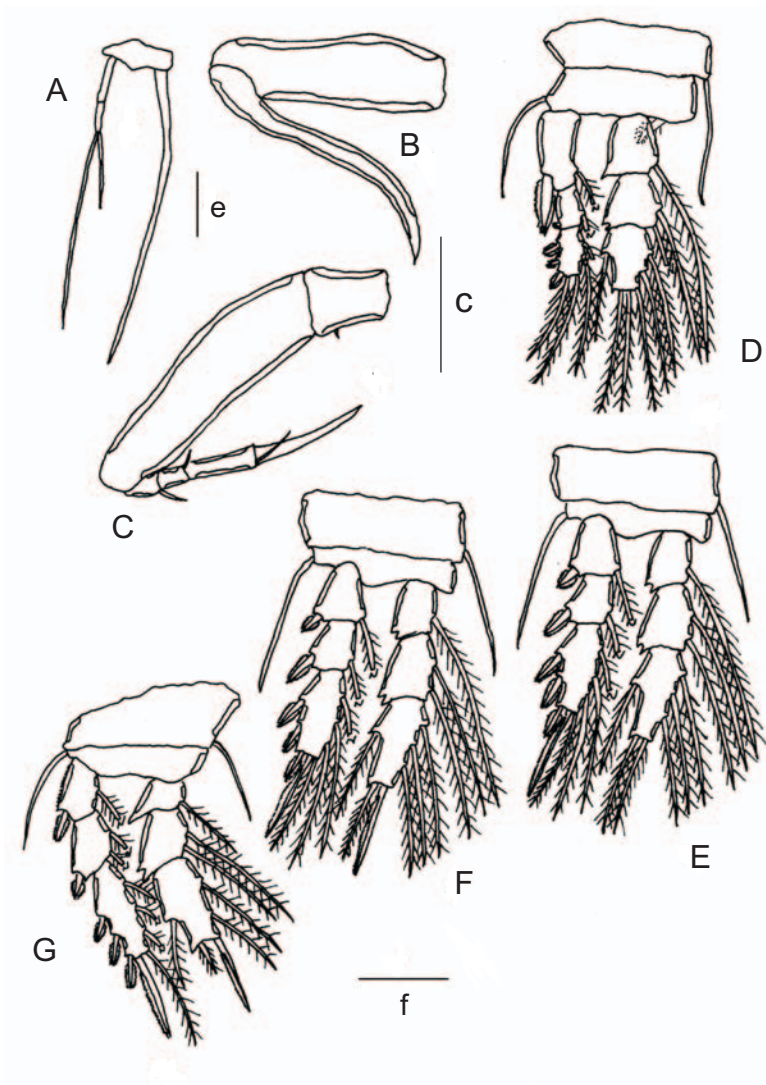
Fig. 2. Asterocheres garridoi sp. nov. Hembra. A: Mandíbula (e); B: Maxila (c); C: Maxilípodo (c); D: Pata 1 (f); E: Pata 2 (f); F: Pata 3 (f) y G: Pata 4 (f). Escala. c,e,f: 0.05 mm.
